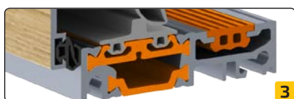
TEPELNĚ IZOLOVANÝ PRÁH
